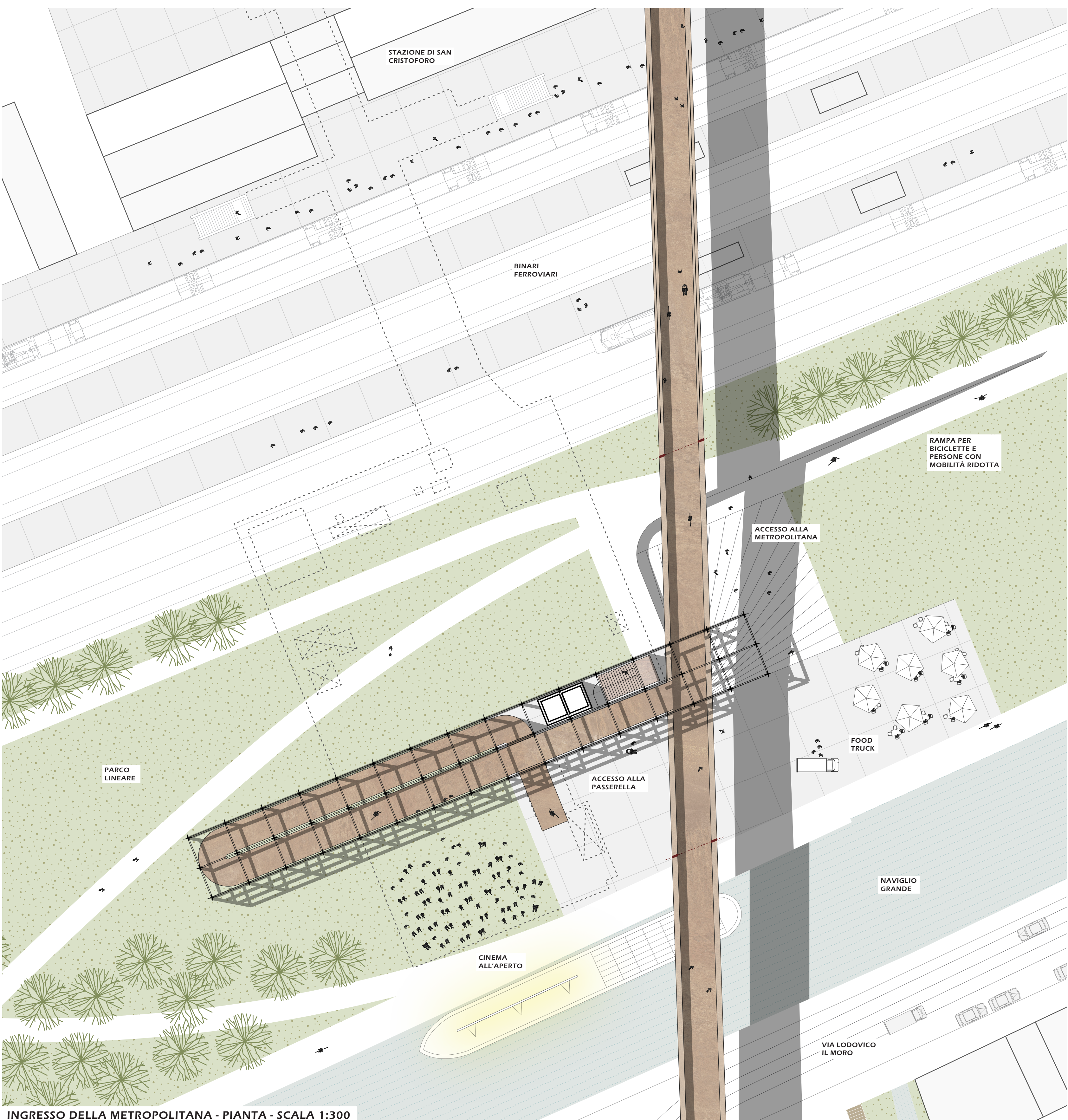
INGRESSO DELLA METROPOLITANA - PIANTA - SCALA 1:300
