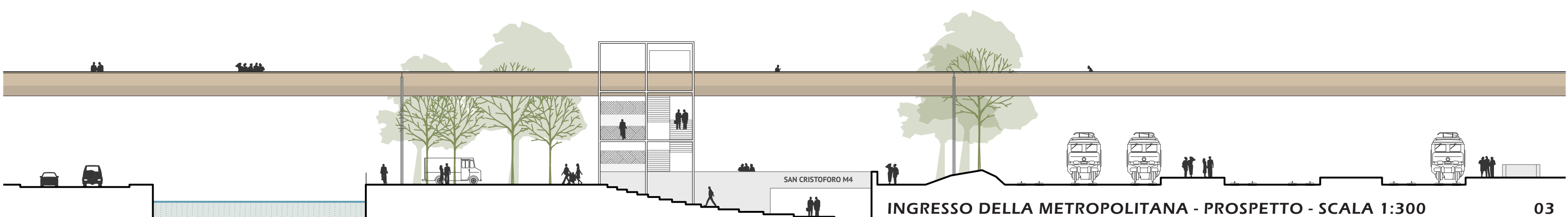
INGRESSO DELLA METROPOLITANA - PROSPETTO - SCALA 1:300
